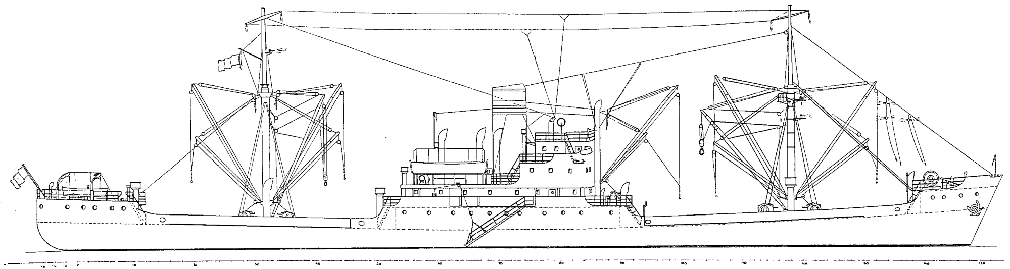
Poopdeck Mittleres Aufbaudeck Bootsdeck Brückendeck Peildeck Backdeck
