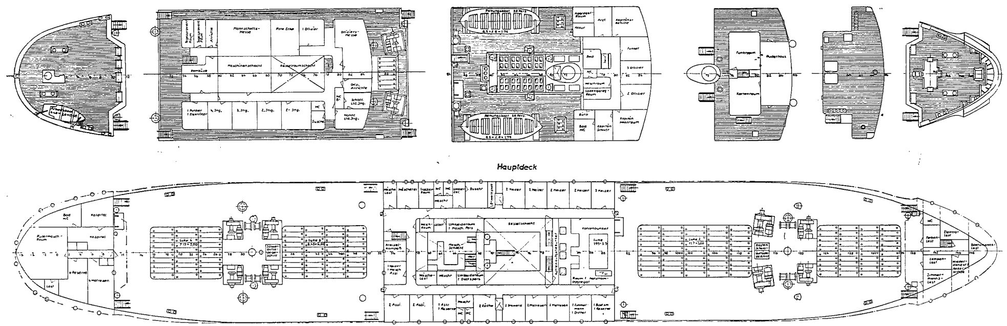
Poopdeck Mittleres Aufbaudeck Bootsdeck Brückendeck Peildeck Backdeck
