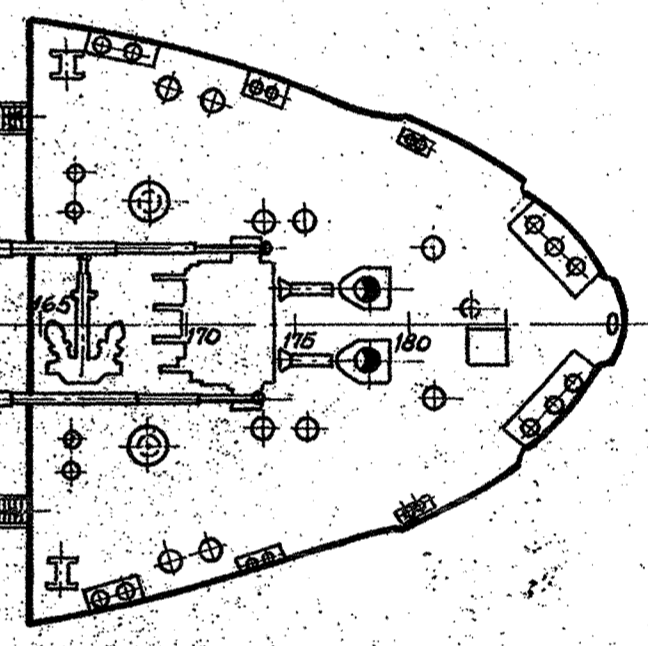
C-Deck
