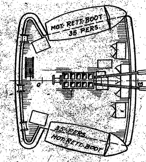
Achternes Deckshausdeck
